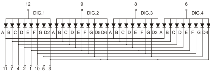
LD4041B
