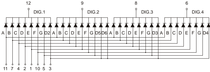
LD4041B
